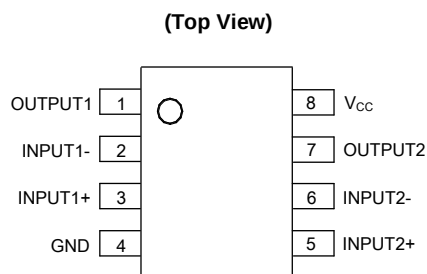
SO-8/TSSOP-8/MSOP-8
